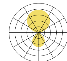
koi-q Pendelleuchte 114lm/W@4000K
