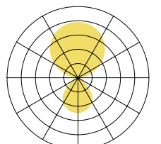
koi-q Stehleuchte/ Tischaufbauleuchte 114lm/W@4000K
