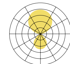
koi-q pendant light 114lm/W@4000K
