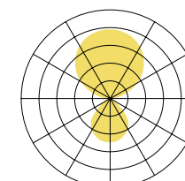
koi-q lampe sur pied/ luminaire de bureau 114lm/W@4000K
