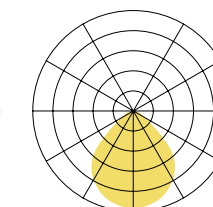
koi-q plafonnier 89lm/W@4000K
