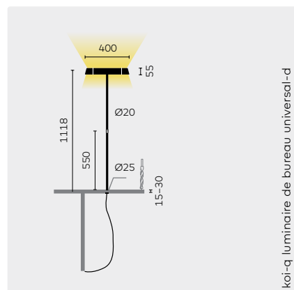
koi-q lampe sur pied
