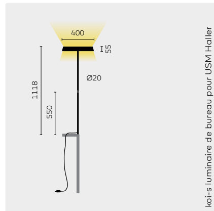
koi-s luminaire de bureau universal-d
