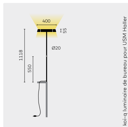
koi-q luminaire de bureau universal-d
